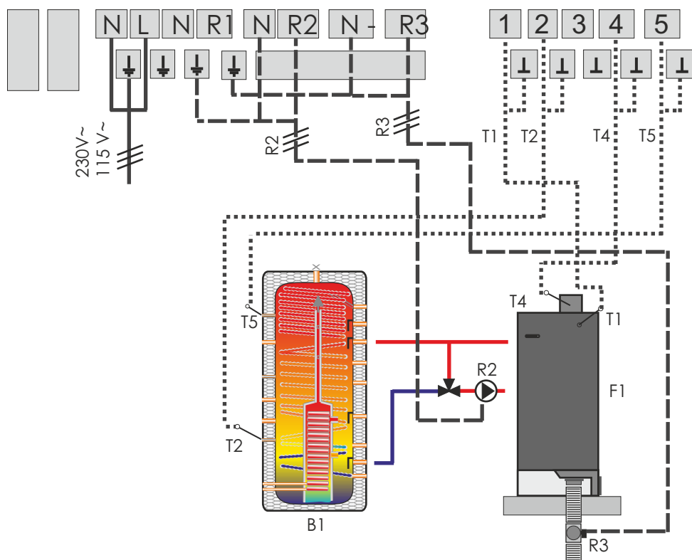
Klemmenplan falls nur die Funktion des Walltherm® wird von der WAL03 geregelt
