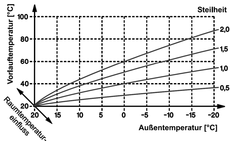
Heizkurve „Steilheit“:
